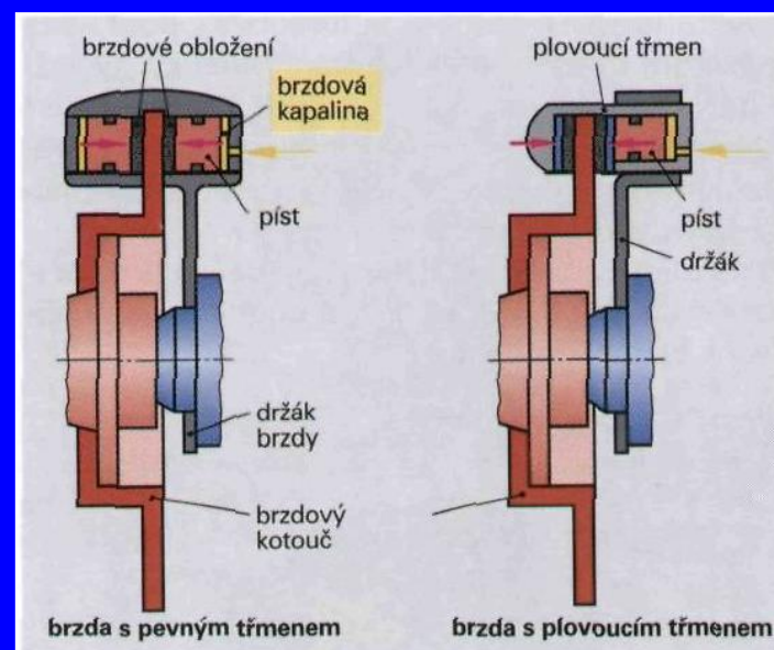
Obr. 2: Dělené kotoučové brzdy
