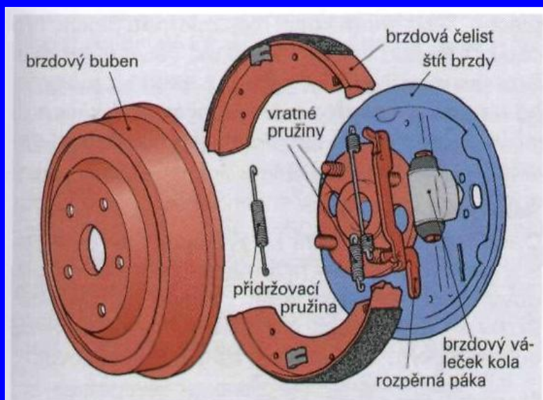
Obr. 1: Části bubnového brzdového ústrojí
